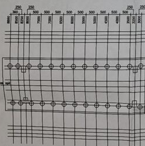
Ankerplan
