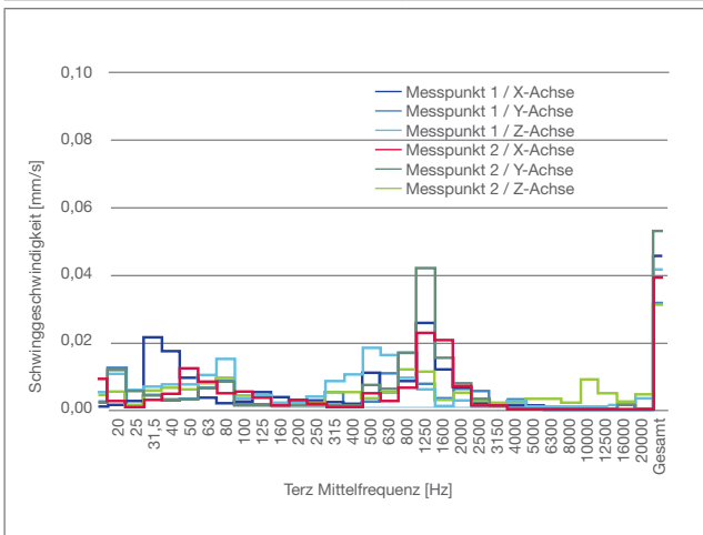
Abbildung 3: Schwingungsgeschwindigkeiten als Funktion der Terz-Mittelfrequenz eines Verdichters. Der Richtwert für den Normalbetrieb laut VDI 2056 liegt bei 4 mm/s. Der QUANTUM-Wert liegt bei rund 0,04 mm/s, also weit darunter.
