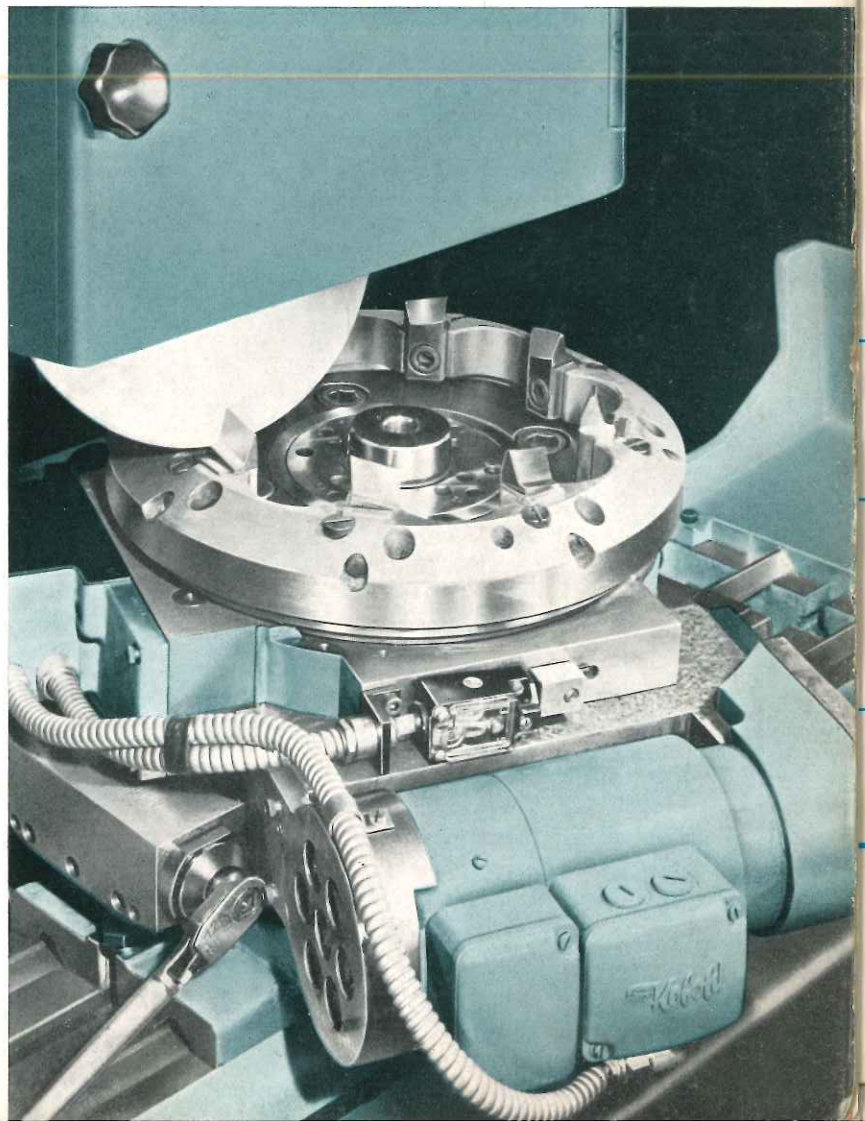
Bild 17: Sonderteileinrichtung ohne Abdeckung
