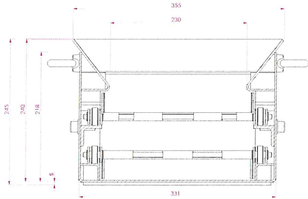
A-A (1 : 1.5)
