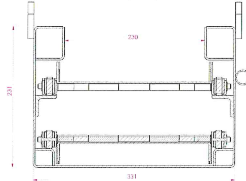
B-B (1 : 1.5)
